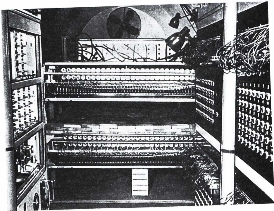
Földalatti mezon-teleszkópok (1958-1986)
