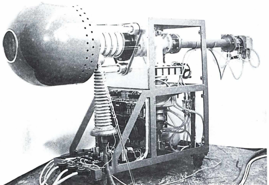
NA-2 neutrongenerátor
