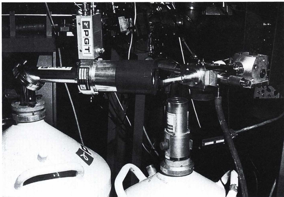
PIXE analitika a Van de Graaff gyorsítónál
