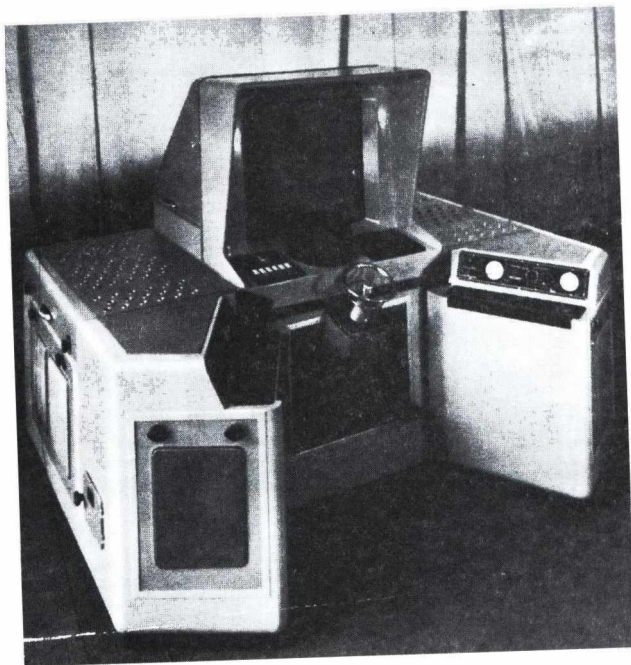
Félautomata buborékkamra felvétel kiértékelő (1959)
