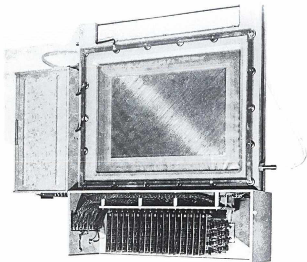
Sokszálas proporcionális kamra (1977)
