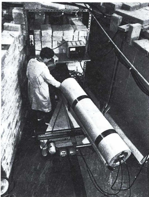
Neutron-diffraktométer
