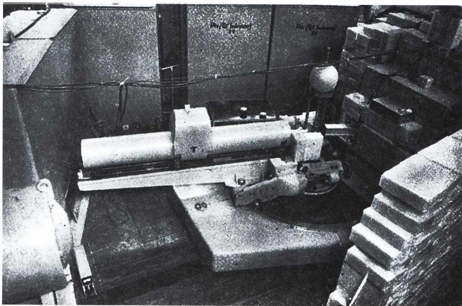
Neutron-diffraktométer
