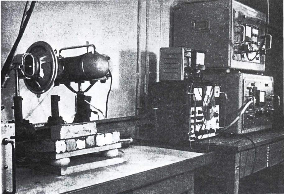
Mössbauer-effektus vizsgálata
