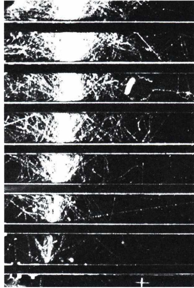
Wilson-kamra felvétel
