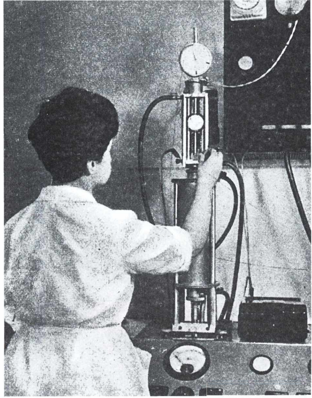
Mössbauer-effektus vizsgálata
