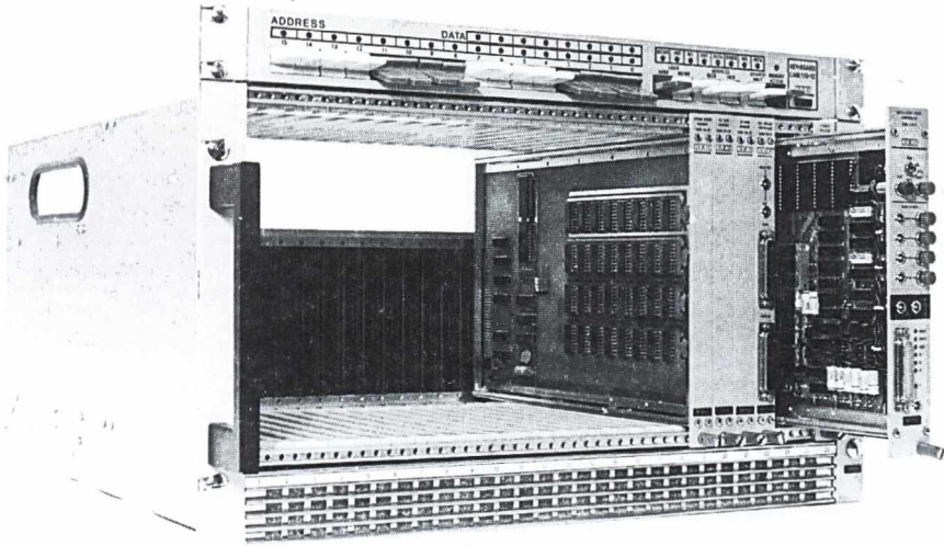
Intelligens CAMAC rendszer (1976)
