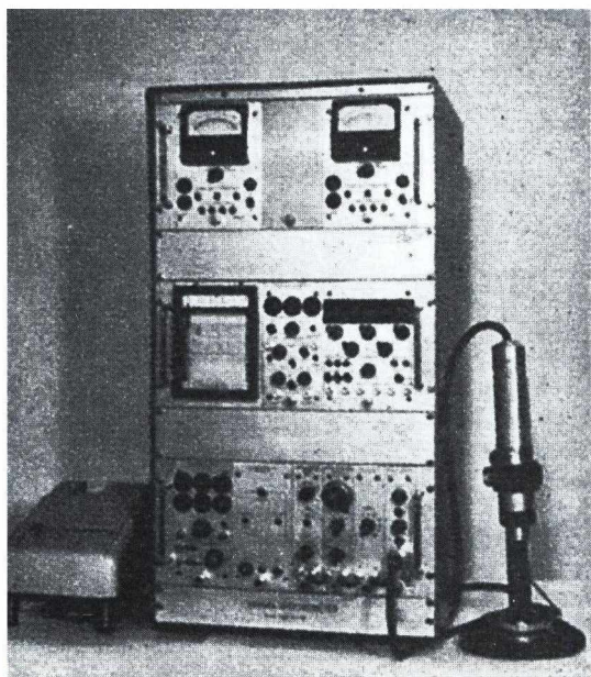
Subrack gamma-spektrométer
