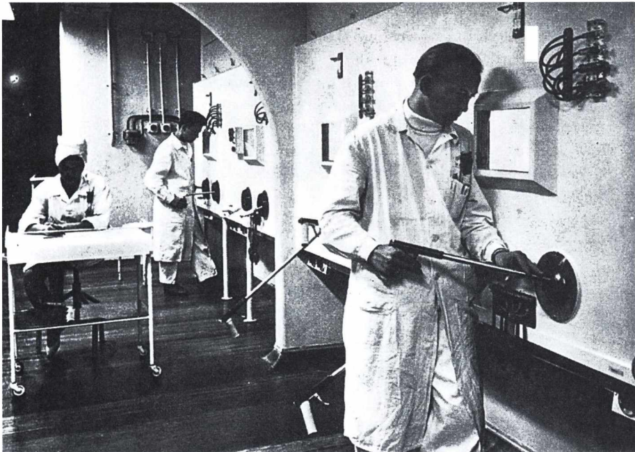
Gamma fülkesor jód-131 gyártásához
