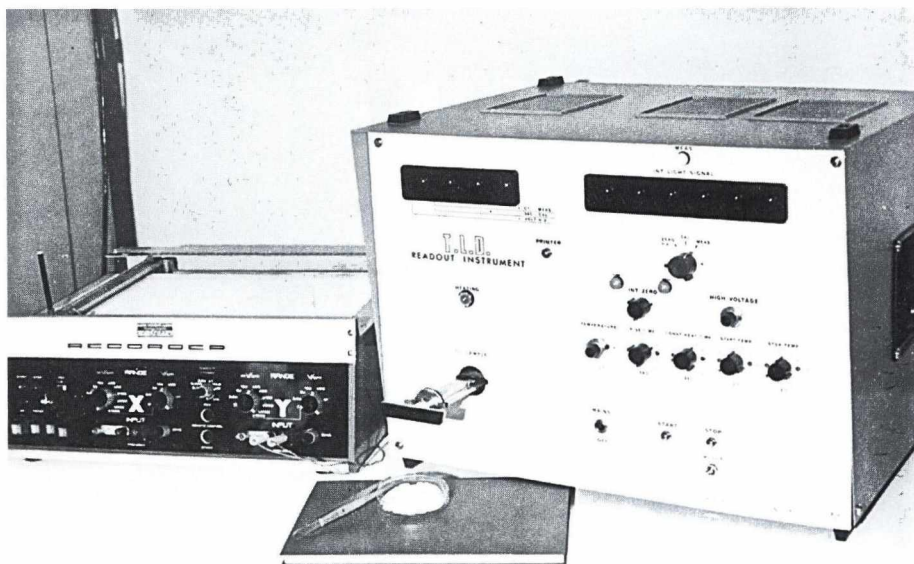
TLD-03 termolumineszcens dózismérő
