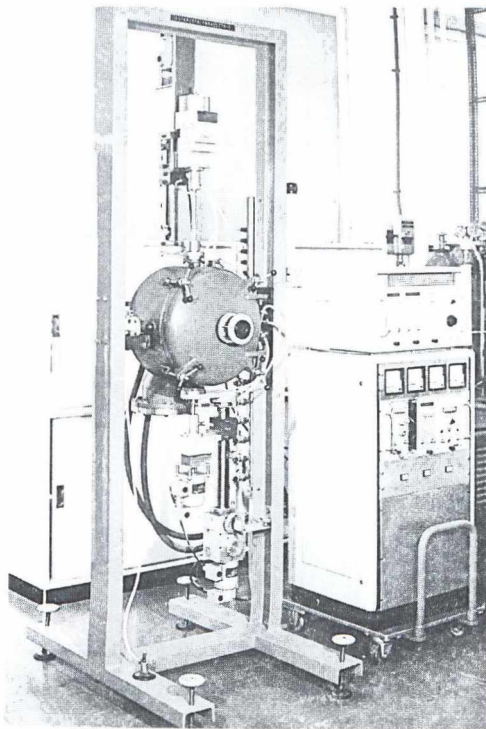
Egykristályok vizsgálata
