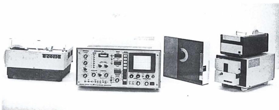
ICA-70 analízátor (1978)
