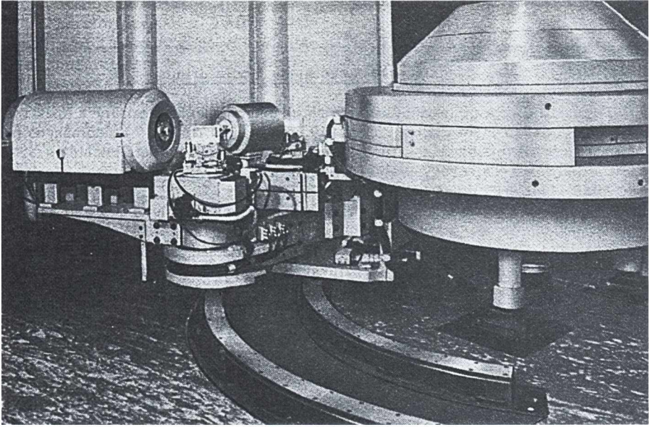
Háromtengelyű kristáljspektrométer
