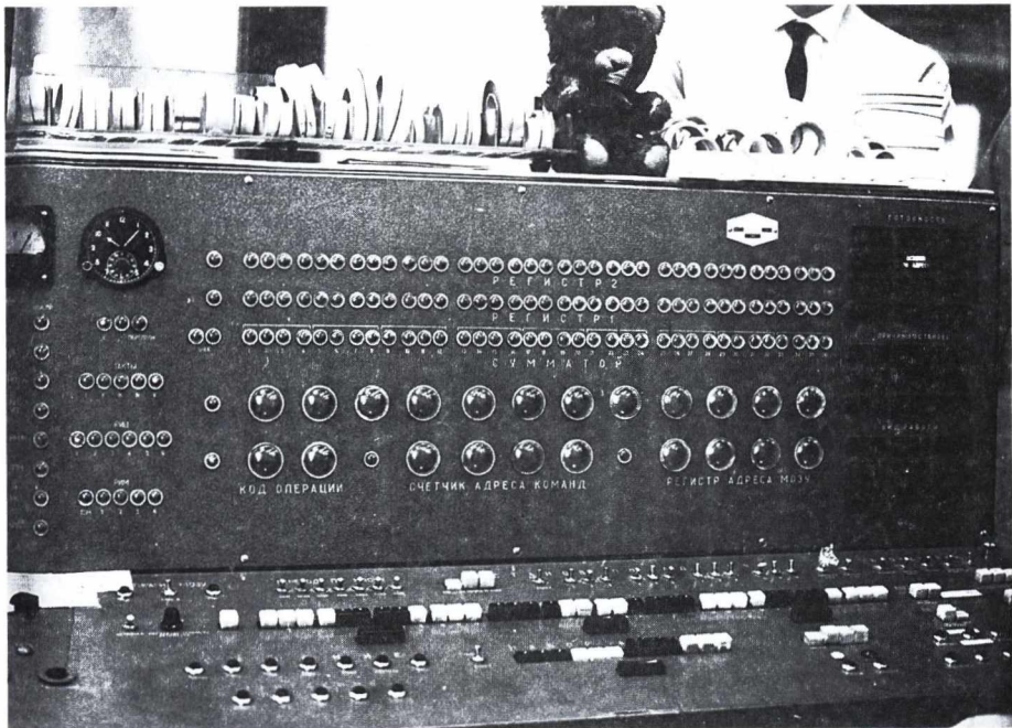
URAL számítógép (1960)
