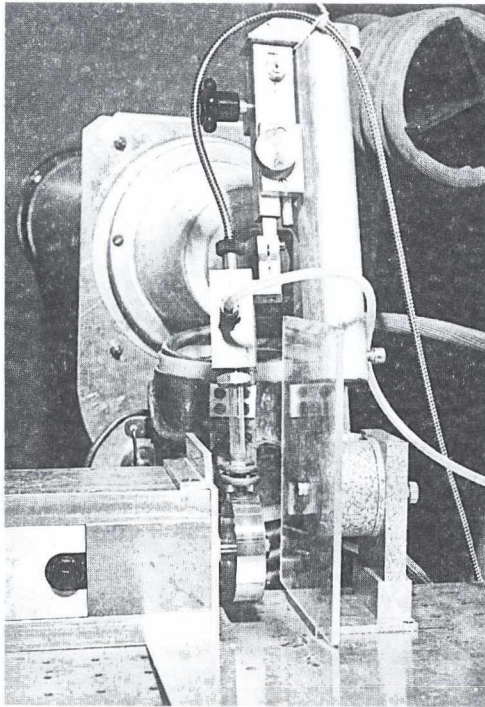
Fémüveg szalag előállítása (1977)
